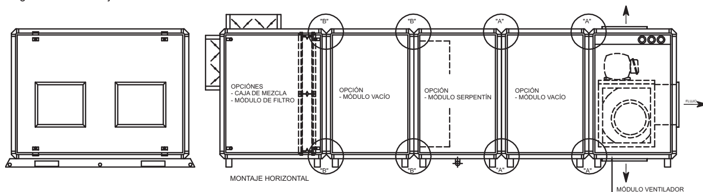
Fig. XVII-20 - Montaje horizontal 02 hasta 40 - WD/WL
