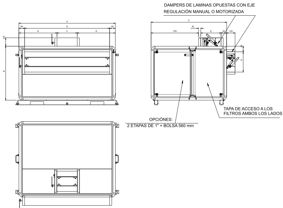
Fig. XVII-08 - Medidas caja de mezcla de los módulos 02 hasta 40 - (2 etapas de 1" + bolsa 560 mm)
