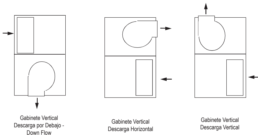
Fig. VII-01 - Opciones de descarga gabinete vertical
