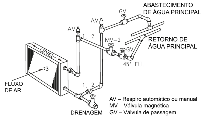
Figura 11 Tubulação típica para serpentina de água
