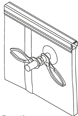
Figura 12 Conexões completamente livres de estresse são essenciais. A tubulação das serpentinas deve ser disposta de modo a facilitar a remoção da serpentina para quaisquer fins de manutenção necessários.
