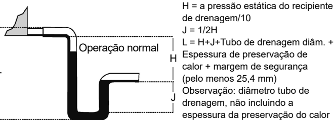
Figura 10 Sifão para módulo sob pressão positiva
