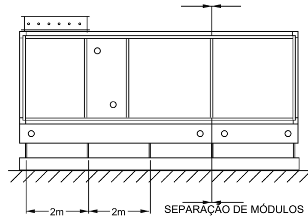
Figura 7 – Base de açoem estrutura metálica da unidade de tratamento de ar
