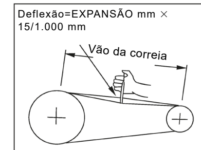
Figura 17 Medição da tensão da correia
