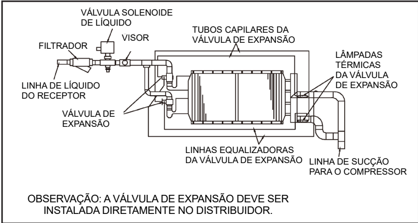
Figura 14 Tubulação típica para serpentina de refrigerante
