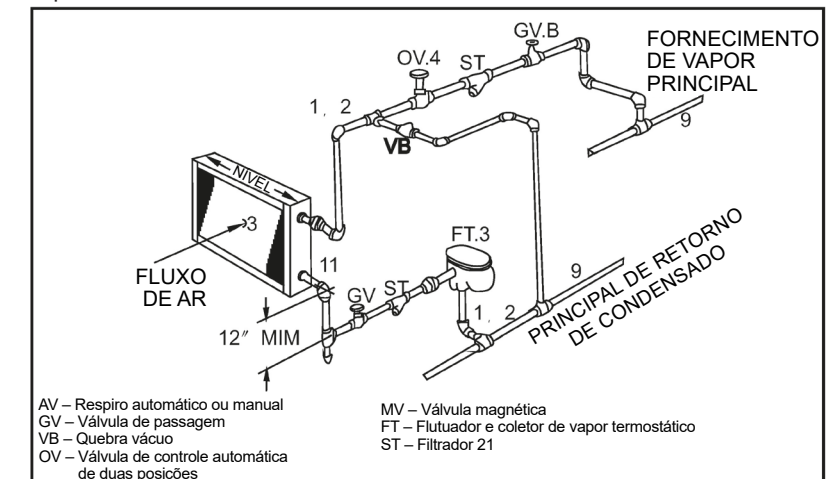
Figura 13 Tubulação típica para serpentina de vapor
