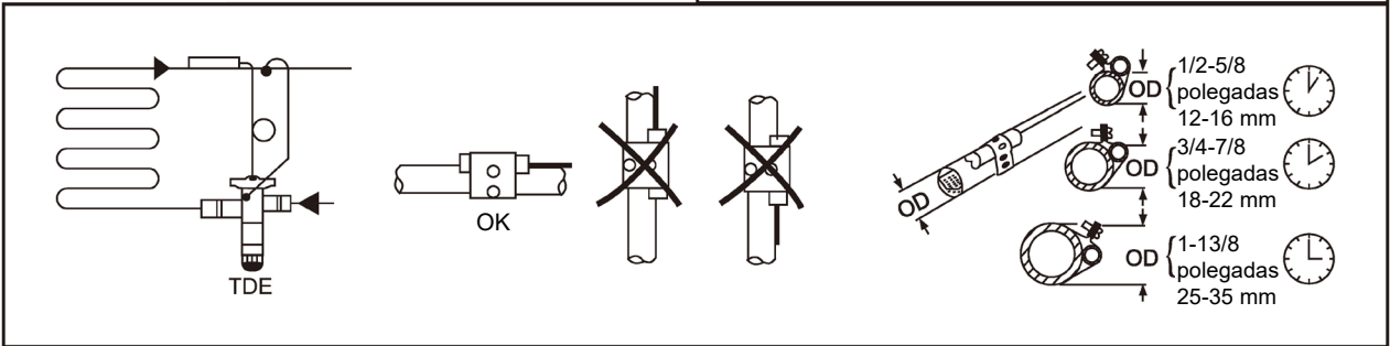
Figura 15 Técnica de solda
