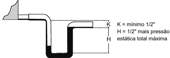
Figura 10 Sifão para módulo sob pressão positiva
