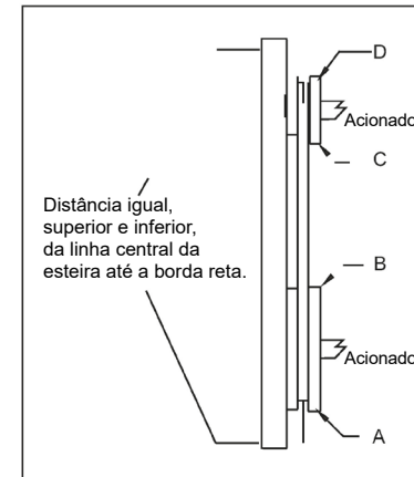
Figura 16 Alinhamento da polia
