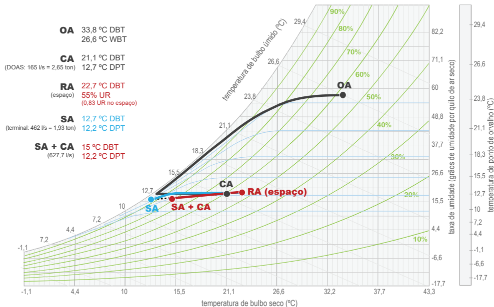
Figura 4. DOAS fornecendo 12,7 °C de ponto de orvalho nas condições do projeto (carga total)
