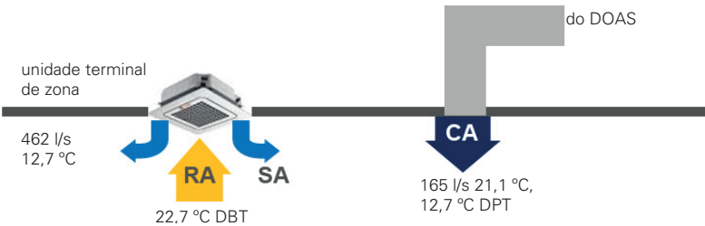
Figura 3. DOAS e unidade terminal em funcionamento nesta sala de aula como exemplo.
